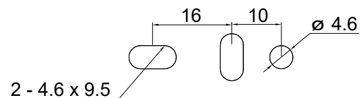
Muster Innenschiene
