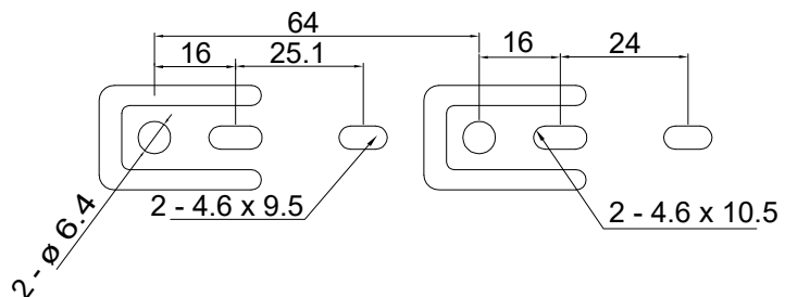
Muster Außenschiene
